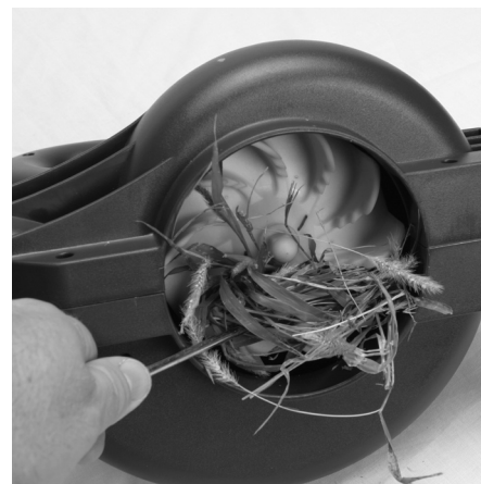
Figure 4-14 : Retrait des débris du rotor
