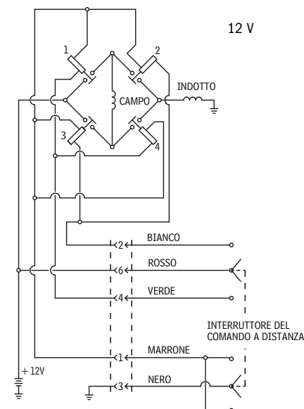
DIAGRAMMA DEL CIRCUITO ELETTRICO
