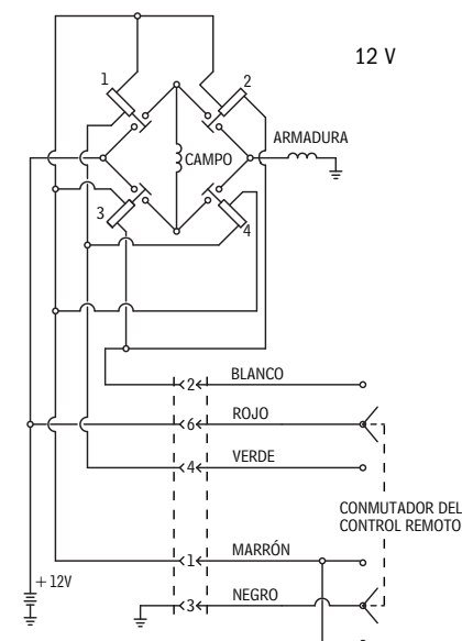
ESQUEMA DEL CIRCUITO ELÉCTRICO
