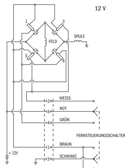
ELEKTRISCHES SCHALTBIELD
