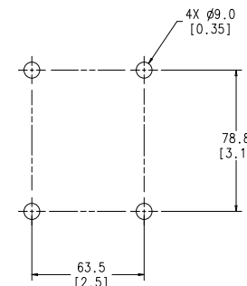
Entraxes de fixation
