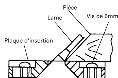
[Coupe de biseau à droite] Fig. 9-c
