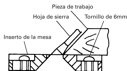
[Corte en ángulo inclinado hacia la derecha] Fig. 9-c
