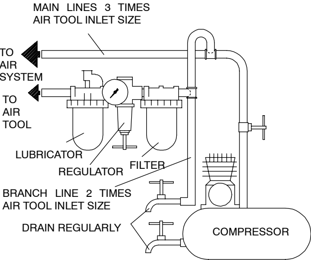
(Dwg. TPD905-1)
